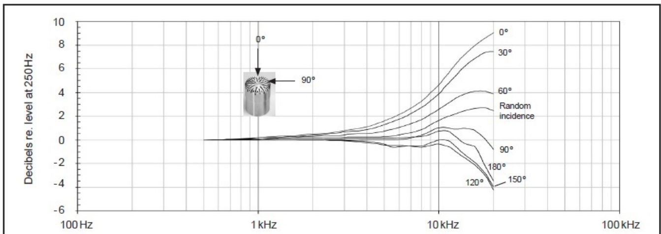
不同入射角下的自由场校正
