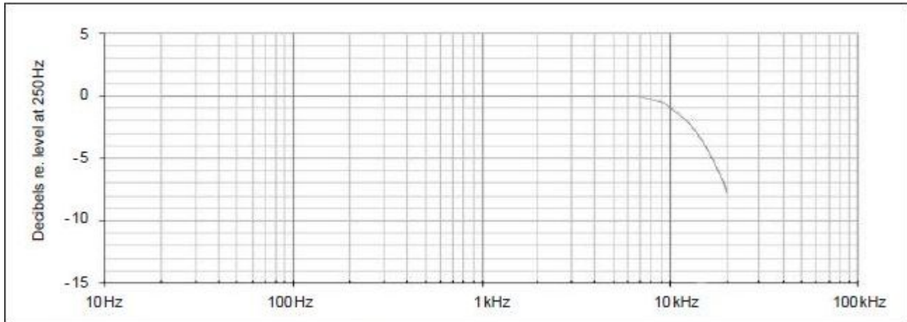
典型频率响应
